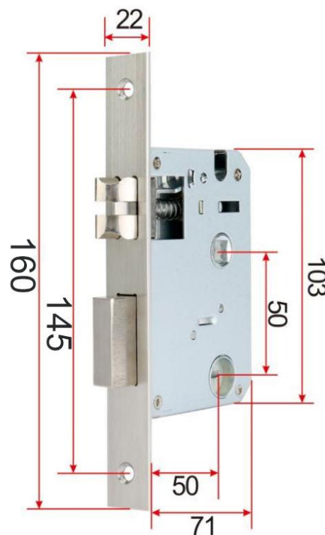
Тип сердцевини 5050
