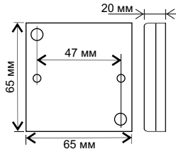
Рис.1 Габариты изделия.
