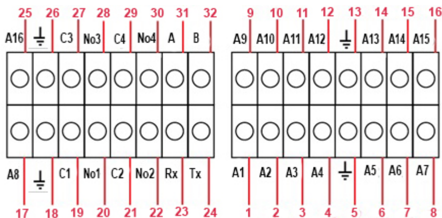
Рис. 1.2.1 «Клеммная колодка регистратора»
