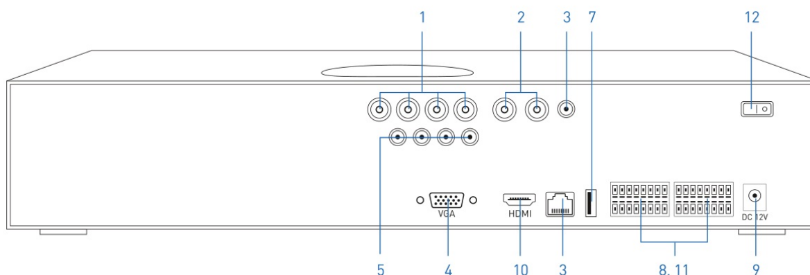
Рис.1.1.1. «Задняя панель регистратора»
